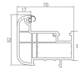
054 Stulp 60mm
