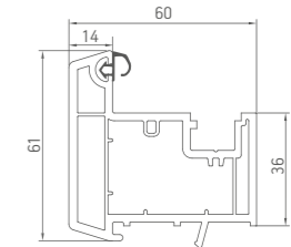
012 Stulp 60mm
