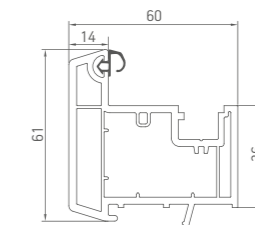
012 Stulp 60 mm
